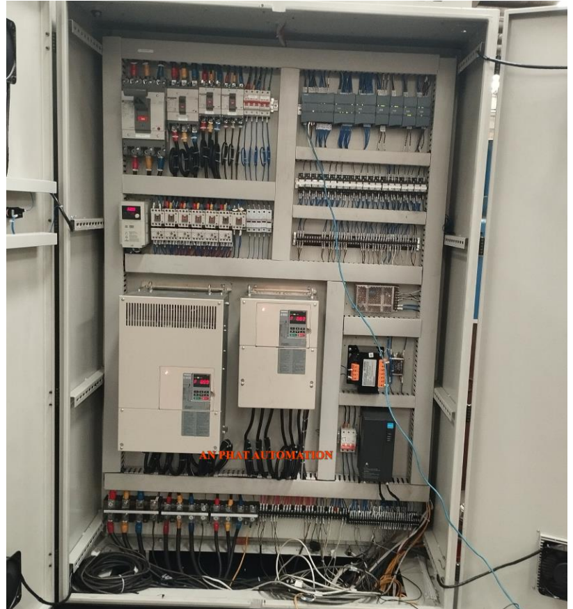
Hệ thống điều khiển cho máy kéo rút – LS Electric cable factory Wire Drawing Machine Control System
