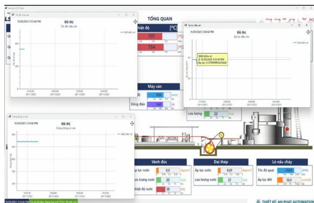
Hệ thống giám sát và thu thập dữ liệu – Nhà máy SX cáp điện LS Vina Supervisory Control and Data Acquisition system – Electric cable factory's LS Vina
