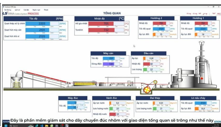
Hệ thống giám sát và thu thập dữ liệu – Nhà máy SX cáp điện LS Vina Supervisory Control and Data Acquisition system – Electric cable factory's LS Vina
