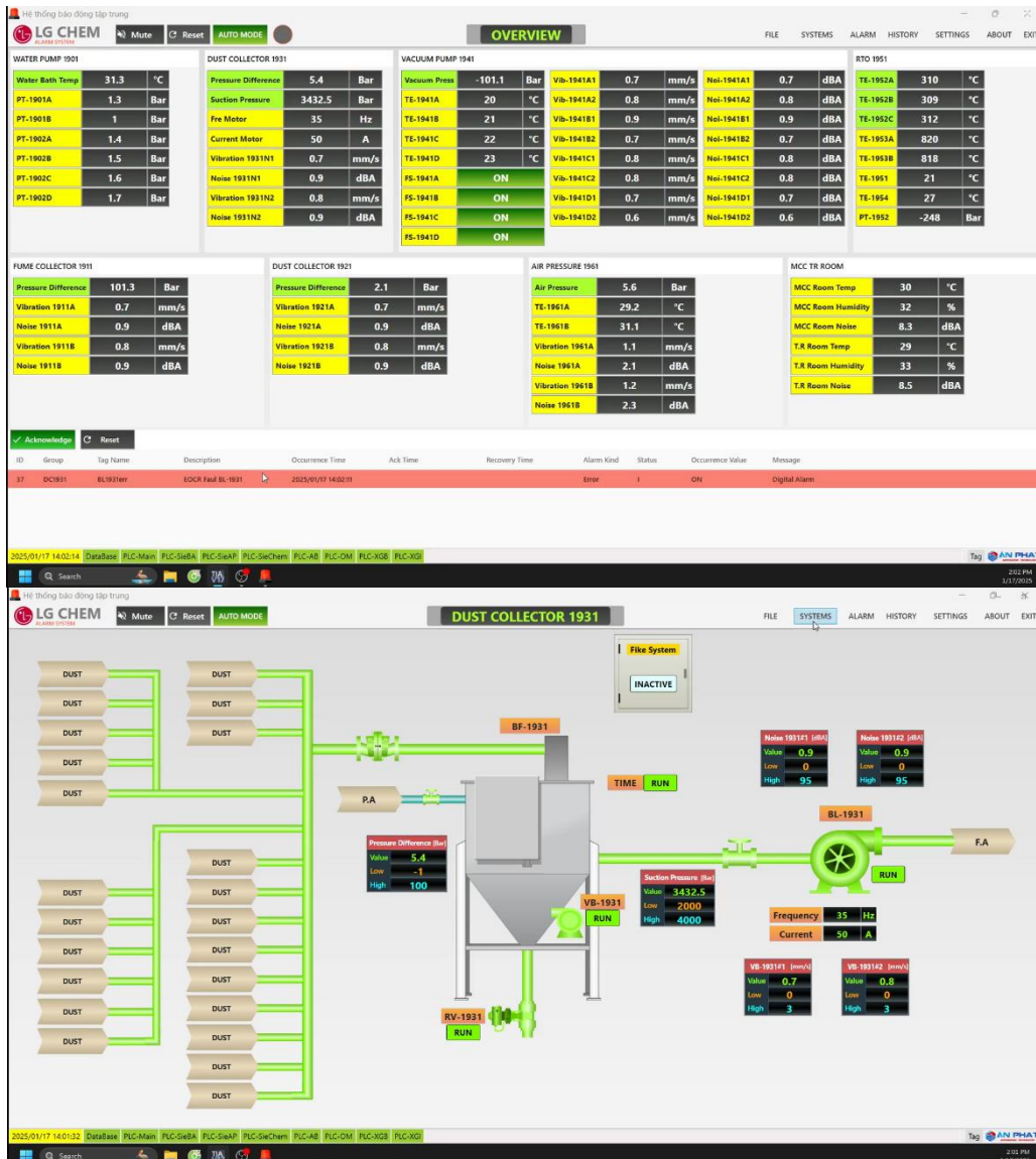
Hệ thống giám sát và thu thập dữ liệu – Nhà máy LG Chem Hải Phòng Supervisory Control and Data Acquisition system – Hai Phong LG Chem factory
