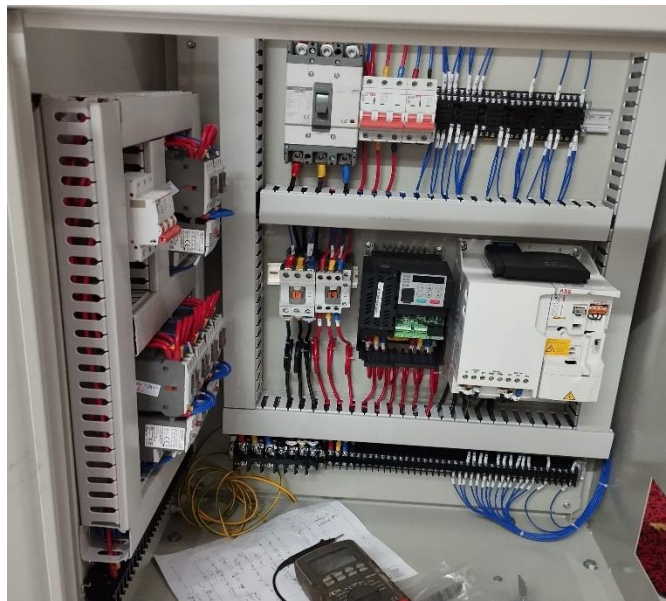
Tủ điều khiển theo yêu cầu Customize control panel
