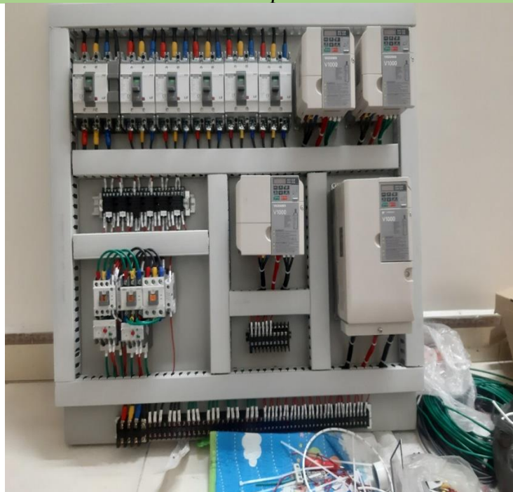
Tủ điều khiển theo yêu cầu Customize control panel
