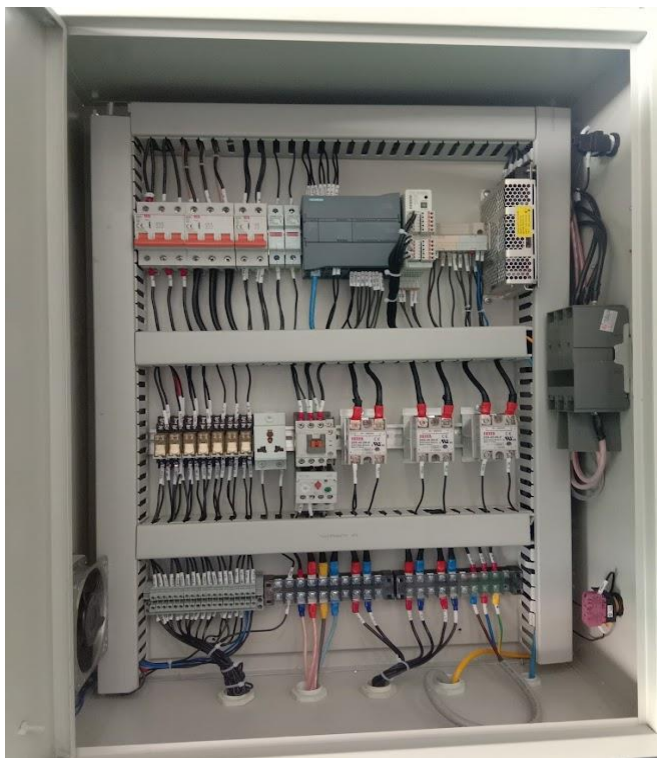
Tủ điều khiển theo yêu cầu - Customize control panel
