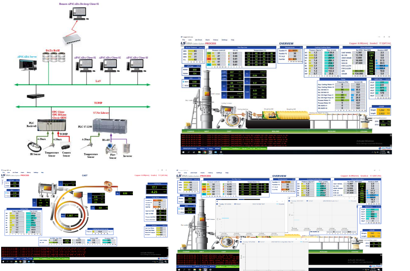
Hệ thống giám sát và thu thập dữ liệu – Nhà máy SX cáp điện LS -Vina Supervisory Control and Data Acquisition system – LS -Vina Electric cable factory
