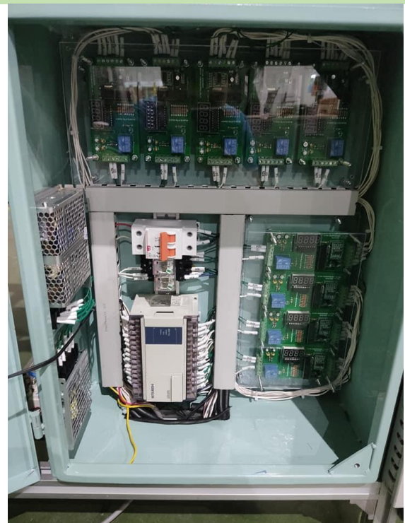
Hệ thống điều khiển máy test vô lăng Tester steering wheel machine control system
