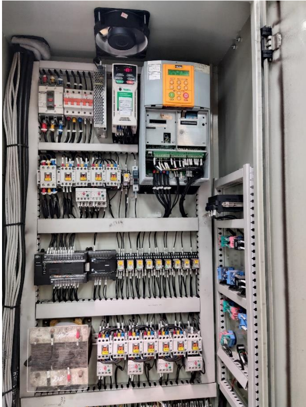
Hệ thống điều khiển máy thu cáp – Nhà máy SX cáp điện Cable winding machine control system – Electric cable factory
